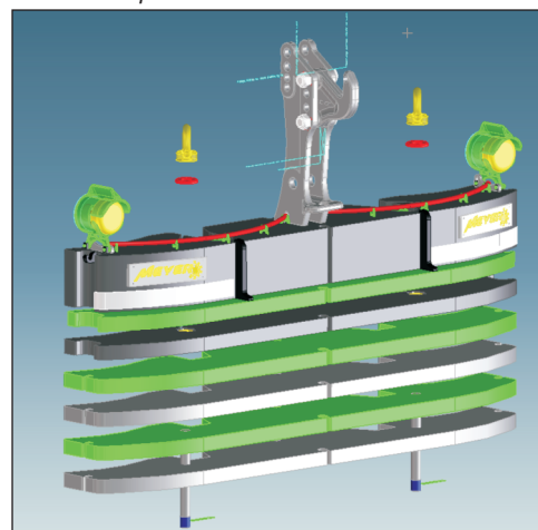
Explosionszeichnung Grundgewicht UF 800 mit 6 Zusatzplatten
